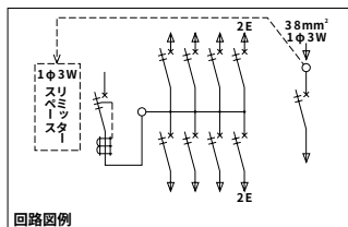
組込例
