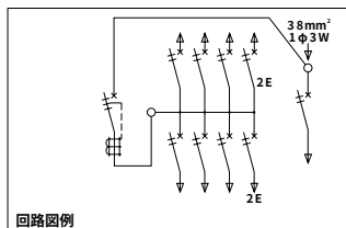
組込例
