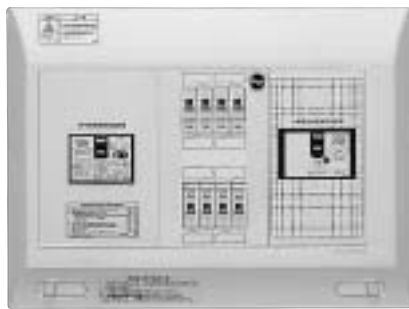
太陽光発電システム対応遮断器組込例
