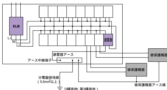
配線用参考図(15回路)
