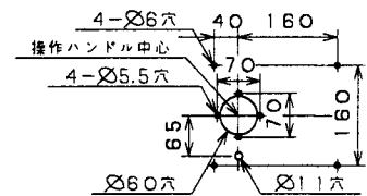
穴明加工図
