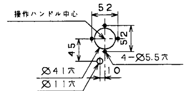
穴明加工図
