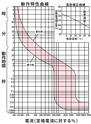
GB-73KA、GBU-73・1KA
