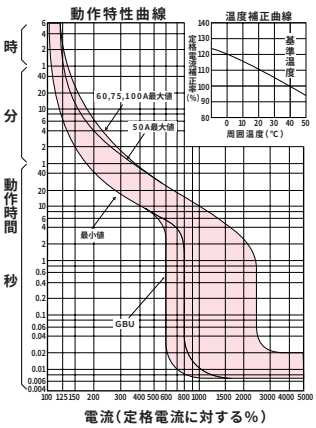
GB-103KA、GBU-103・1KA、GBU-103KA
