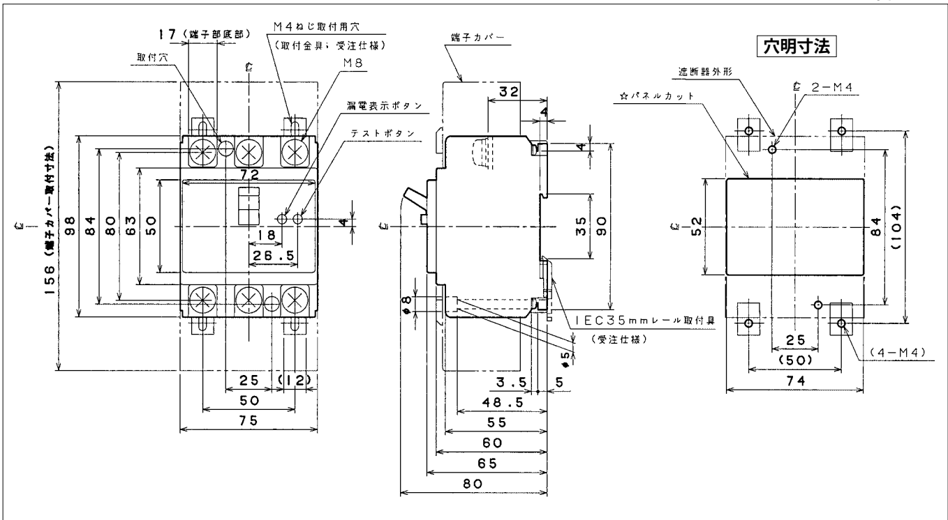
GB-73KA、GBU-73・1KA
