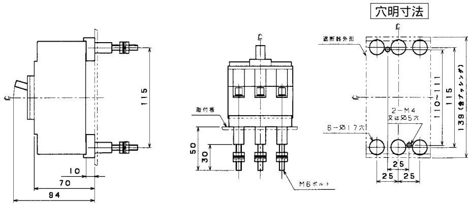
裏面形 (SD)
