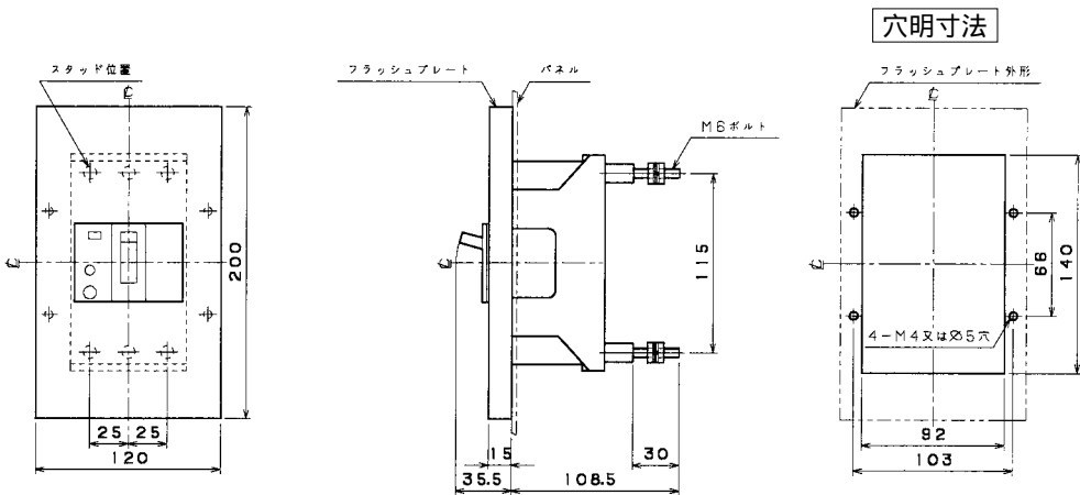
埋込形 (FP)
