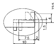
ロックレバー部(B部)詳細
