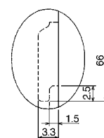
取付部(A部)詳細
