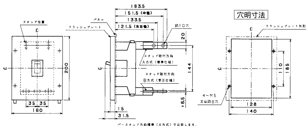
埋込形 (FP)
