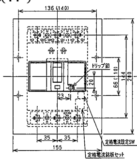
埋込形 (FP)
