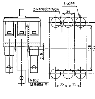
穴明寸法
