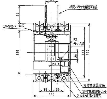
裏面形 (SD)
