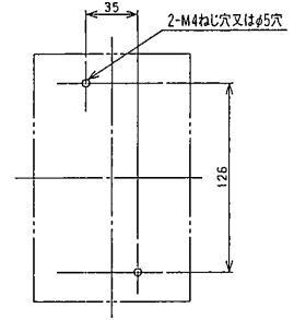
穴明寸法
