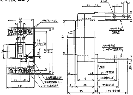
裏面形 (SD)
