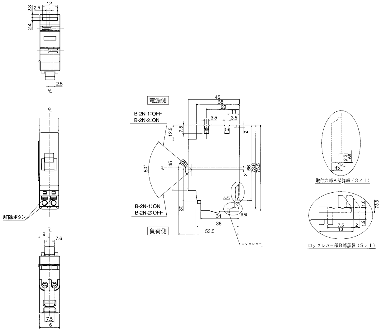
B-2N-1・B-2N-2(15A・20A)
