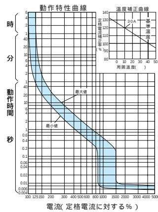
B-2N-1・B-2N-2(30A)
