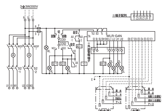
TNG4AW-SU (自動交互同時運転用)
