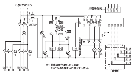
TNG3A (自動交互運転用)
