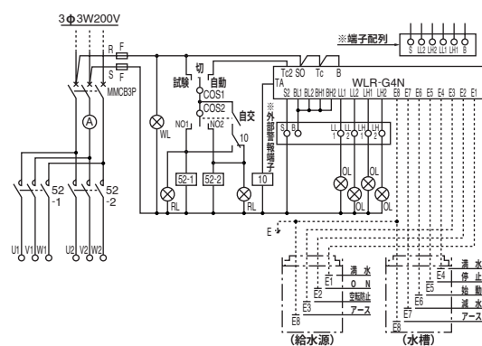
TNG4A-SU (自動交互運転用)
