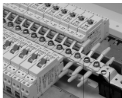
分岐接続バー 母線
