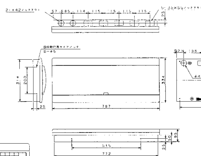
埋込形
