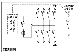
回路図例
