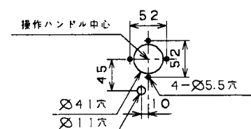
穴明加工図
