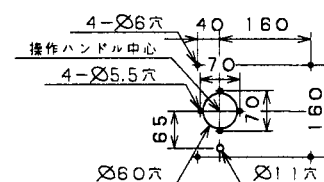
穴明加工図
