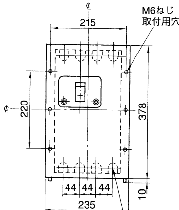
埋込形 (FP)
