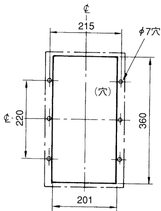
穴明寸法
