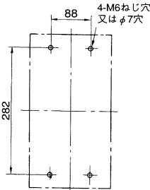
せん孔図
