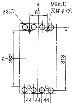
せん孔図
