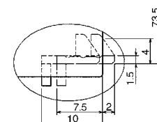
ロックレバー部(B部)詳細
