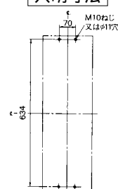
穴明寸法
