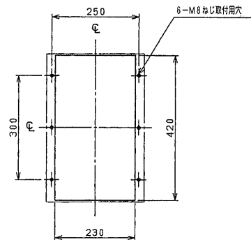
穴明寸法
