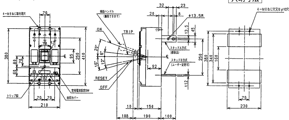
穴明寸法
