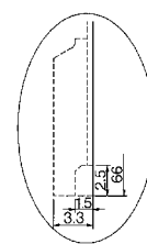
取付穴部A部詳細 (3/1)
