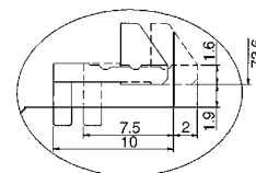
ロックレバー部B部詳細 (3/1)
