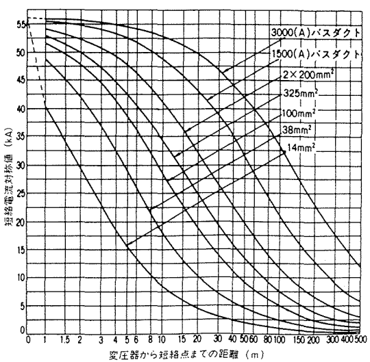
付図16 三相変圧器容量750kVA、二次電圧200V
