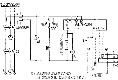
TNG2（単独自動運転用）
