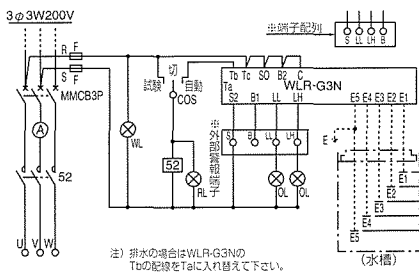
TNG3（単独自動運転用）
