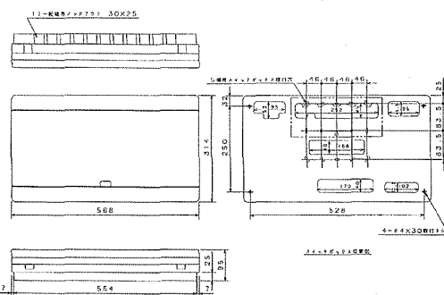
露出・半埋込形
