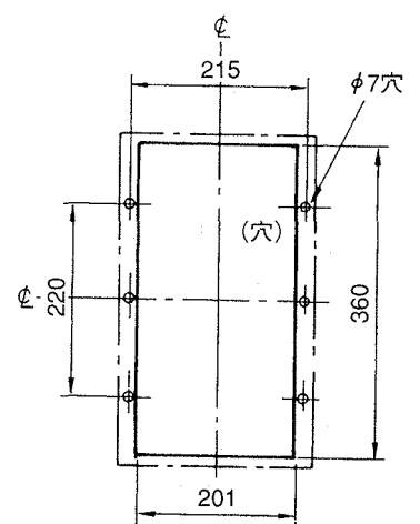
穴明寸法
