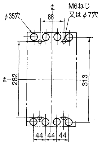
せん孔図
