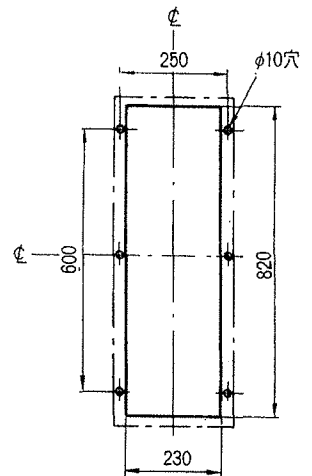
穴明寸法
