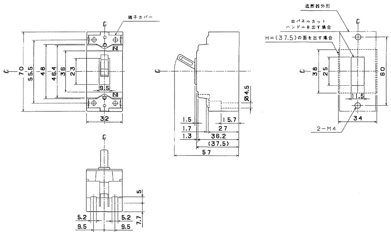
穴明寸法
