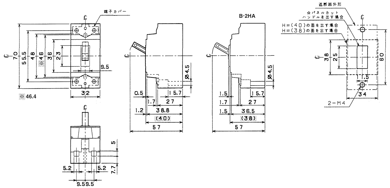
穴明寸法
