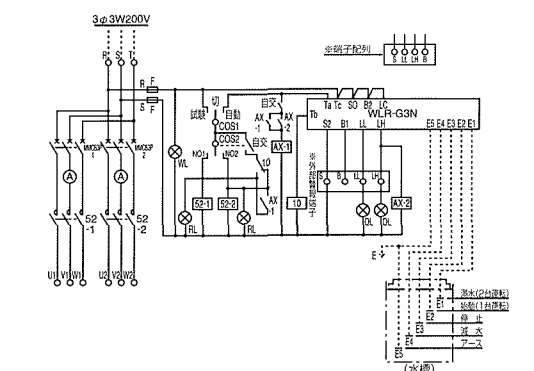
TNG3AW (自動交互同時運転用)
