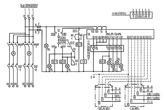
TNG4AW-SU (自動交互同時運転用)
