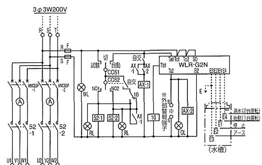
TNG2AW (自動交互同時運転用)
