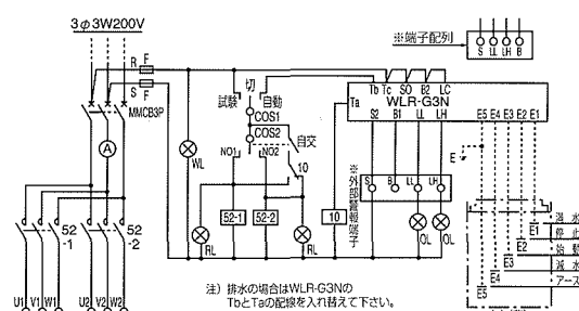
TNG3A (自動交互運転用)
