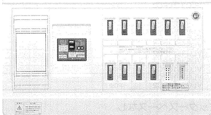
ピーク電流音声警報器 (PW-1) 組込例
