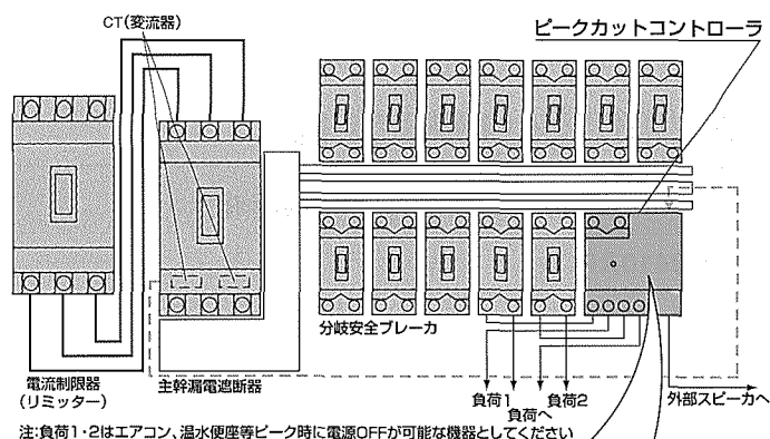
ピークカットコントローラ PC-3 (レベル表示付き)
