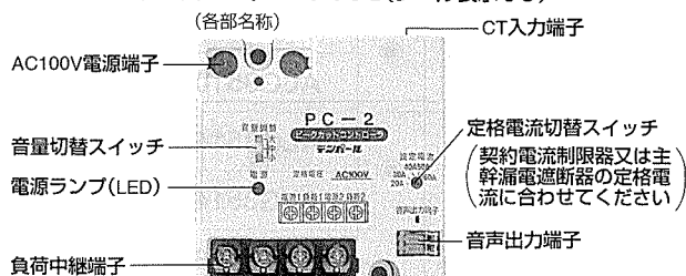
ピークカットコントローラ PC-2 (レベル表示なし)
