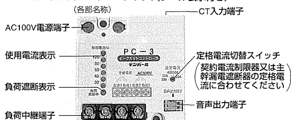
ピークカットコントローラ PC-3 (レベル表示付き)
