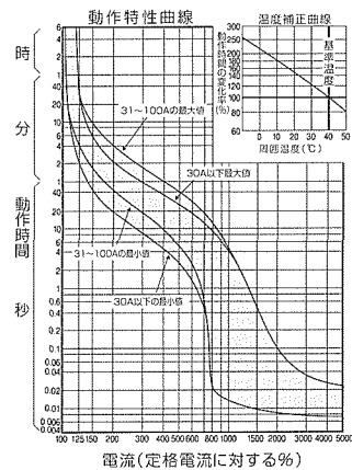
36 GBU-53・1J, BU-53・1J
