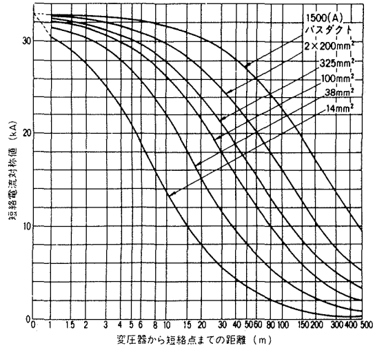
付図19 三相変圧器容量1000kVA、二次電圧415V
