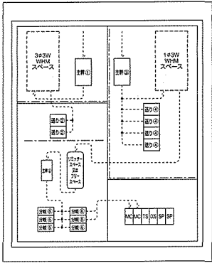
回路図(A)
