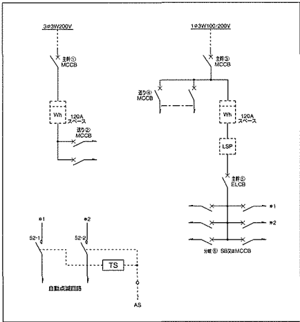
■回路図(A)
