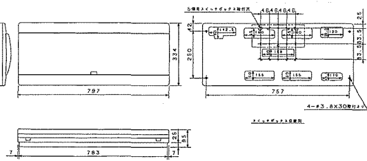
露出・半埋込形
