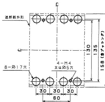
穴明寸法
