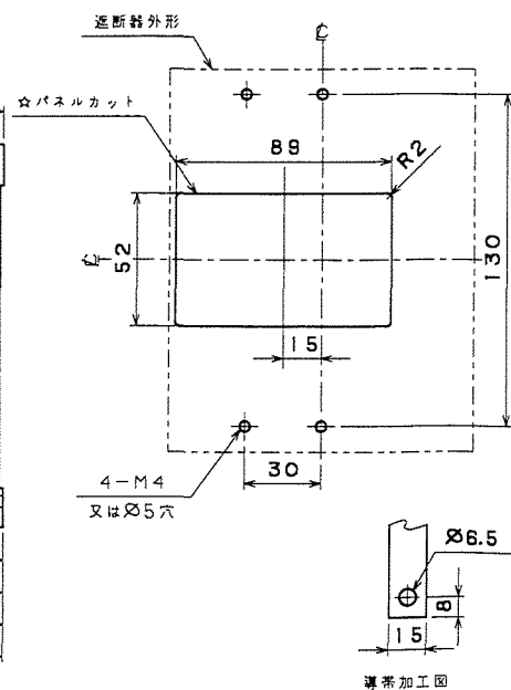
穴明寸法
