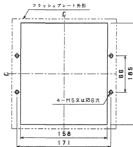
穴明寸法
