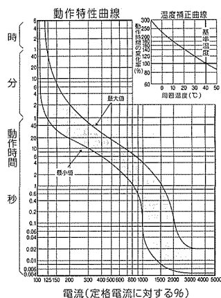
28 GB-73KA, GBU-73・1KA
