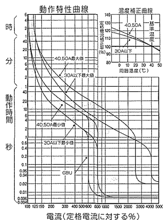
29 GB-103KA, GBU-103・1KA, BU-103・1KA
