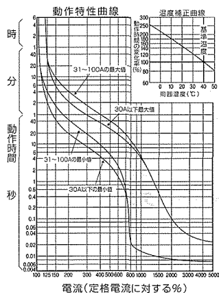
35 GBU-53・1J, BU-53・1J
