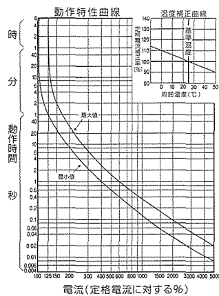
5 B-33EA
