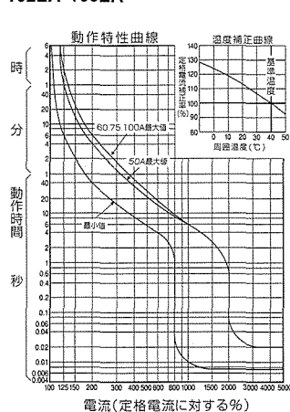
11 B-252E・253E
