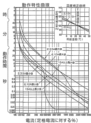
4 B-32EB
