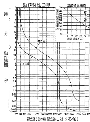
6 B-52EB, B-53EA
