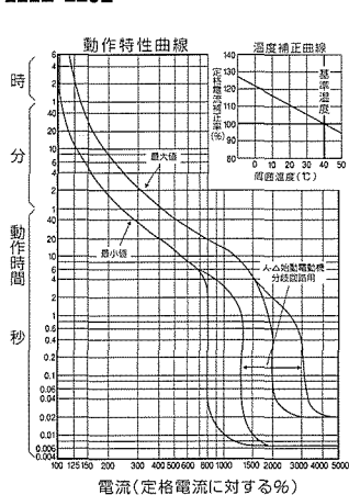
10 B-222E・223E
