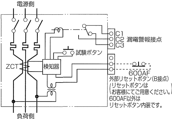
■外部リセット仕様内部回路図(600AF)
