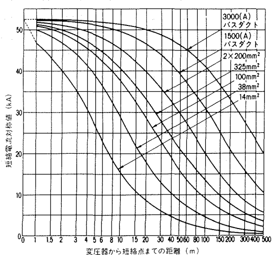
付図23 三相変圧器容量2000kVA、二次電圧415V
