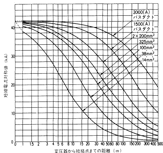
付図21 三相変圧器容量1500kVA、二次電圧415V
