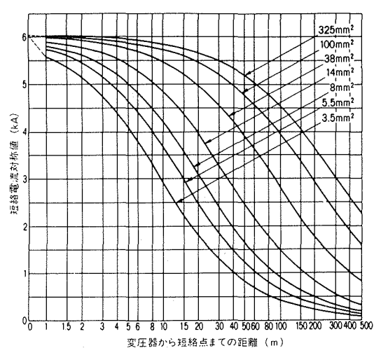
付図7 三相変圧器容量100kVA、二次電圧415V
