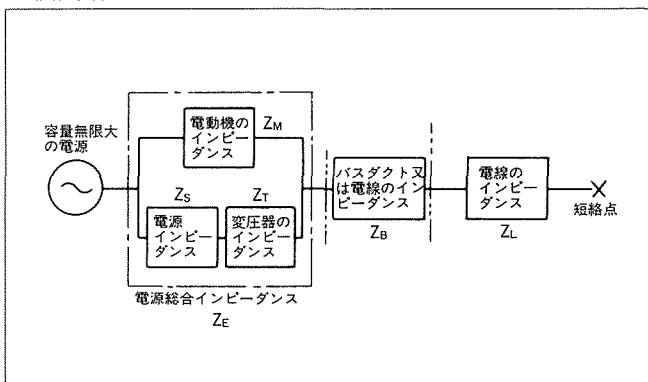
等価回路
