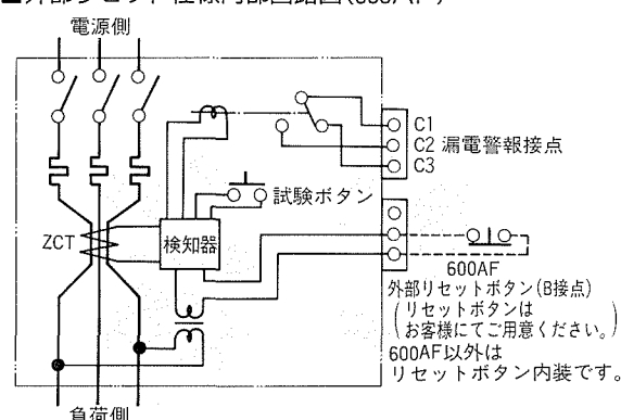
■外部リセット仕様内部回路図(600AF)
