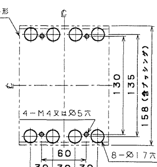
穴明寸法
