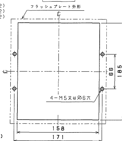
穴明寸法
