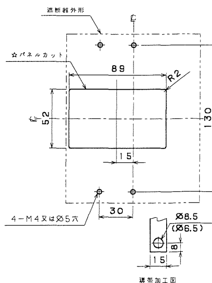
穴明寸法
