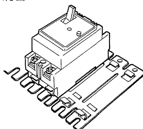
② 取付台
