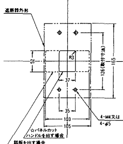
穴明寸法
