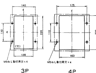
穴明寸法
