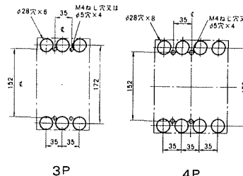
穴明寸法
