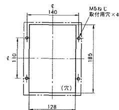
穴明寸法
