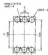
穴明寸法
