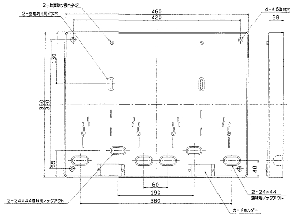
77 2P-WE (フットカバー付)
