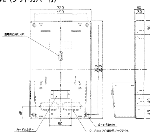
77 2P-WE (フットカバー付)
