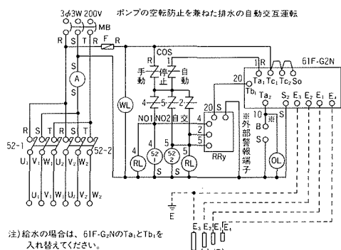
TNG4A (自動交互運転用)
