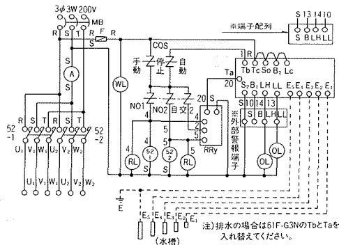
TNG4A-SU (自動交互運転用)
