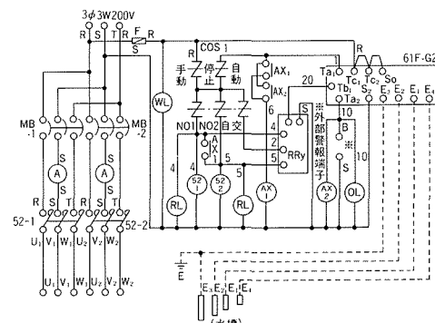
TNG4AW (自動交互同時運転用)
