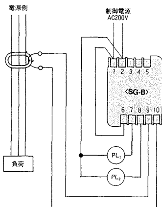
【C】警報装置を取付ける場合 SG-Bが動作した時PL 2 が点灯し動作しない時はPL 1 が点灯します。
