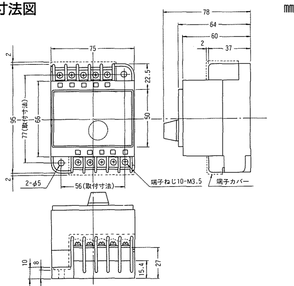
外形寸法図
