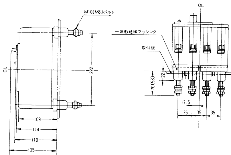
裏面形(SD)
